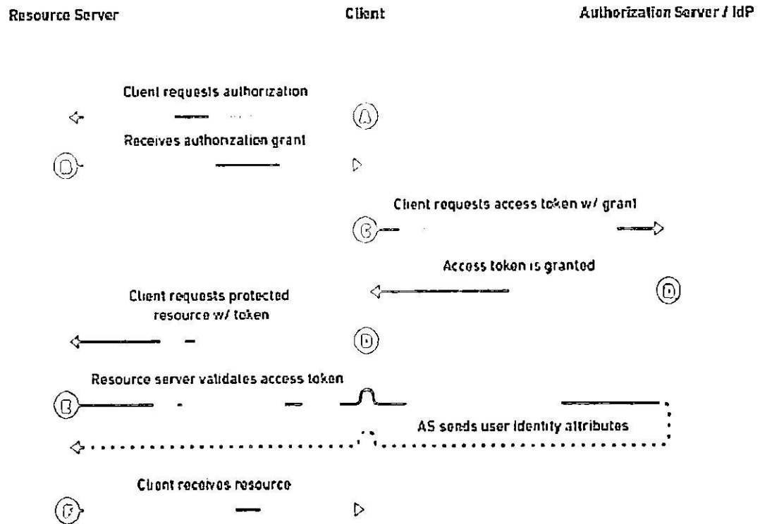
Hình 2: Sơ đồ cơ chế OpenID Connect
